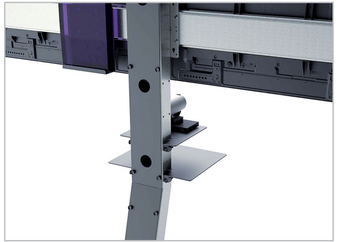
Edelstahlsäule mit innenliegender Kabelführung
